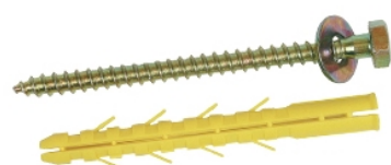
Cheville sabot de charpente
